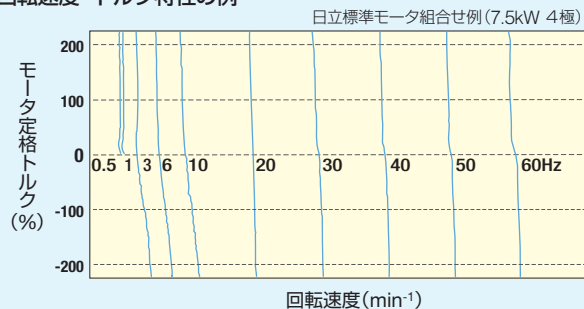
回転速度・トルク特性の例
