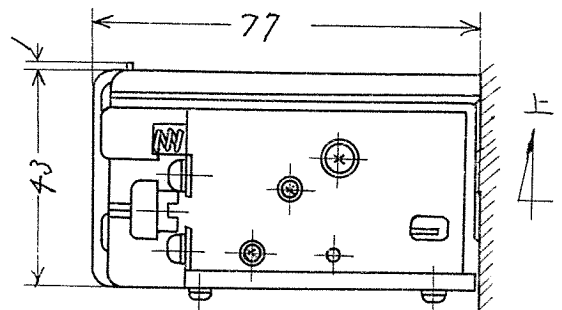
取付状態
