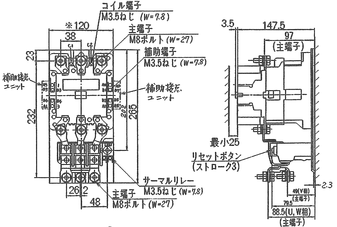
取付状態
