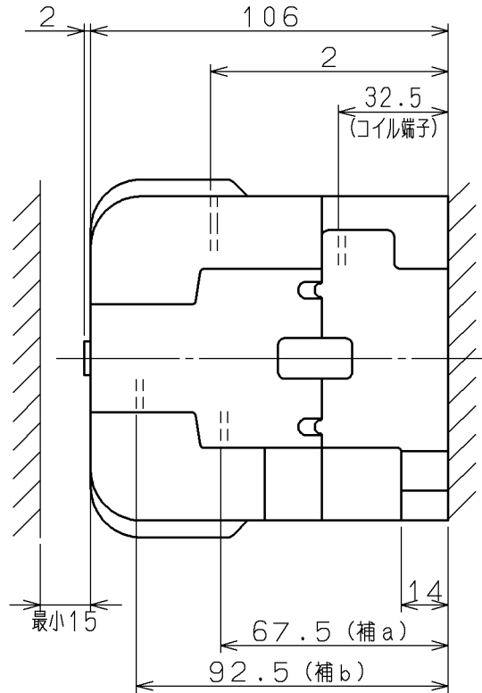
取付状態
