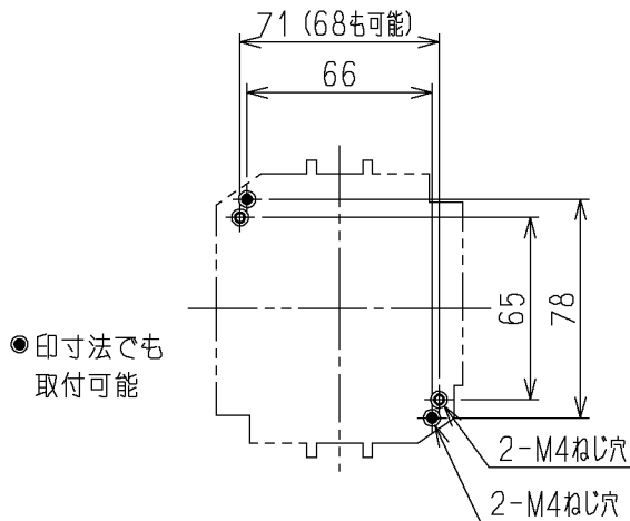
せん孔図
