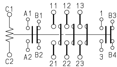
接点構成
