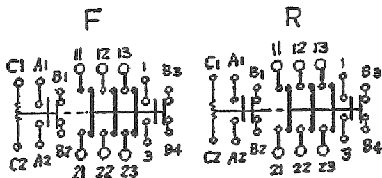
接点構成
