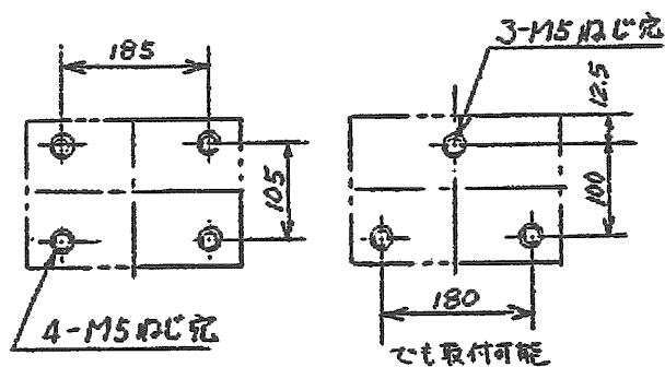
せん孔図
