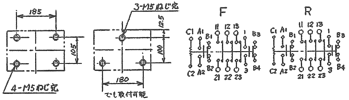
接点構成
