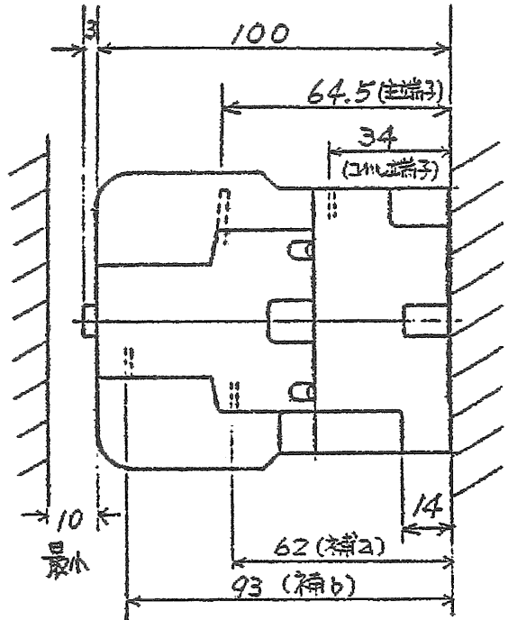
取付状態
