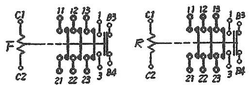
接点構成
