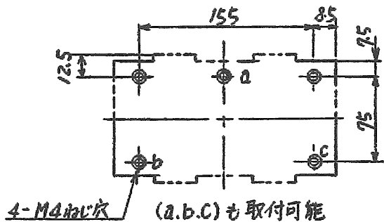
せん孔図
