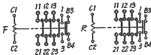
接点構成
