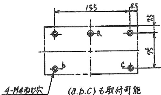
せん孔図
