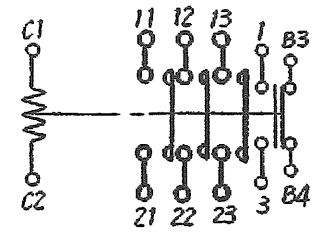
接点構成
