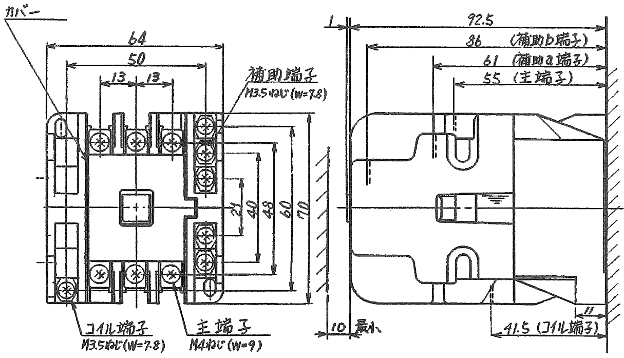
取付状態
