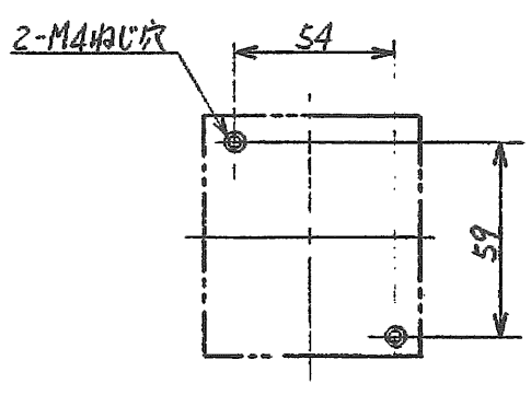
54×56, 54×60も取付可能 せん孔図
