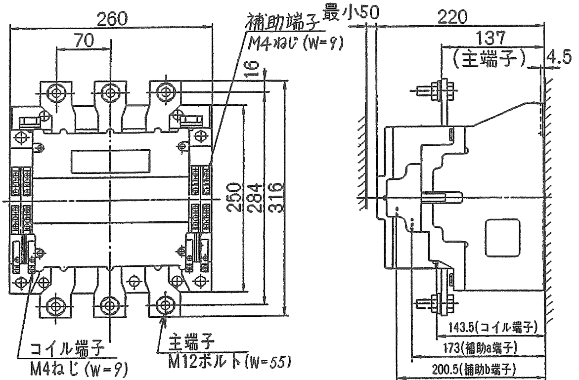
取付状態
