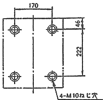
せん孔図
