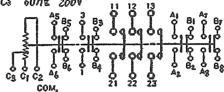
接点構成
