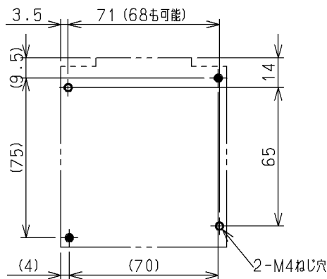
せん孔図
