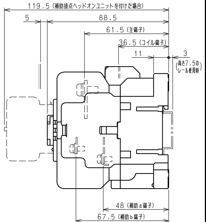
取付状態
