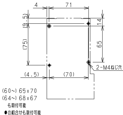
せん孔図
