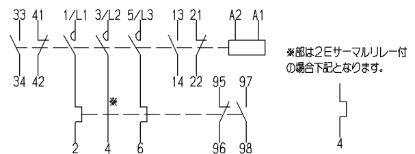
接点配置
