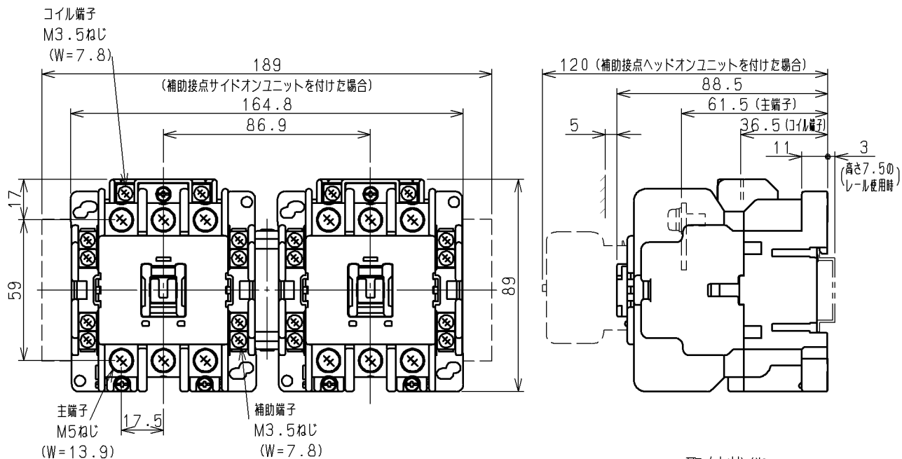
取付状態
