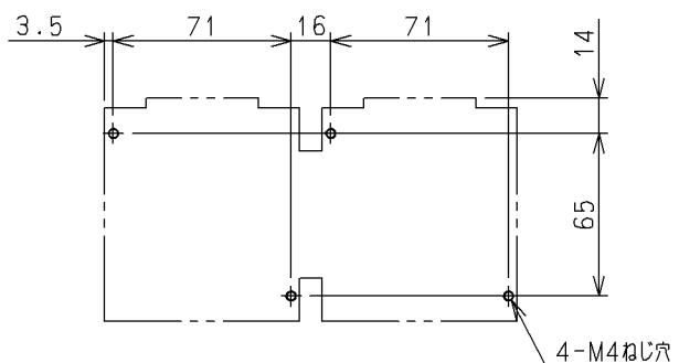
せん孔図
