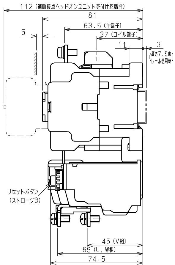
取付状態
