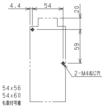
せん孔図
