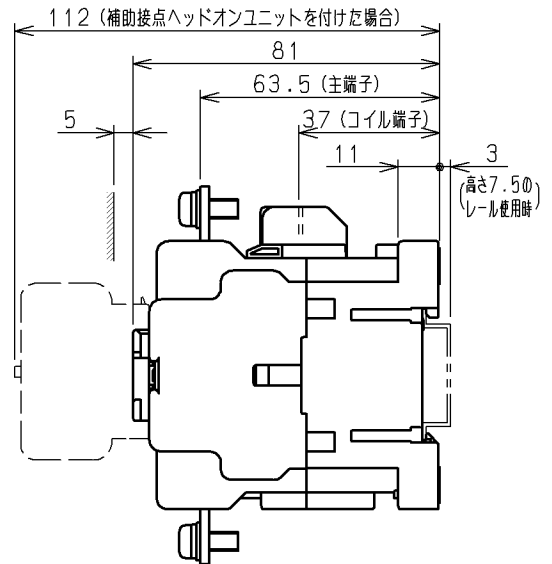
取付状態
