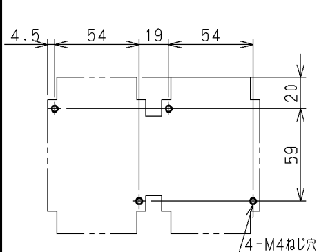
せん孔図
