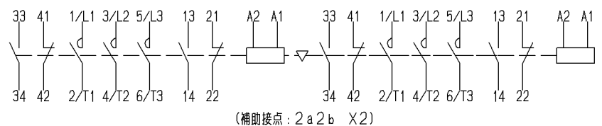
接点配置
