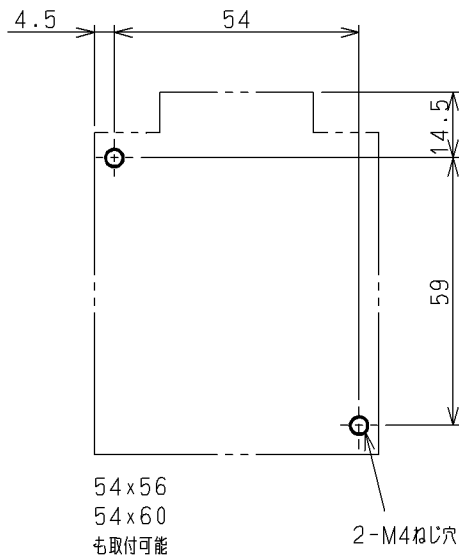
せん孔図
