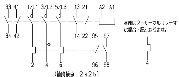
接点配置
