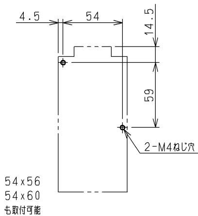
せん孔図
