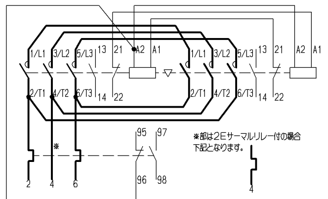
接続図
