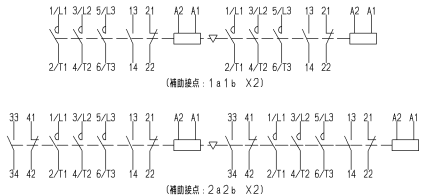
接点配置
