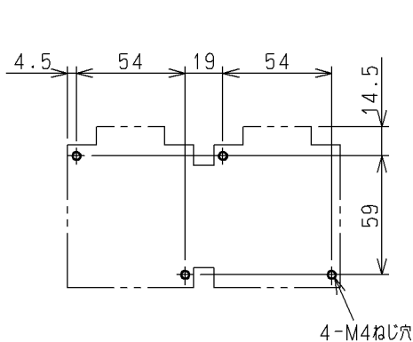
せん孔図
