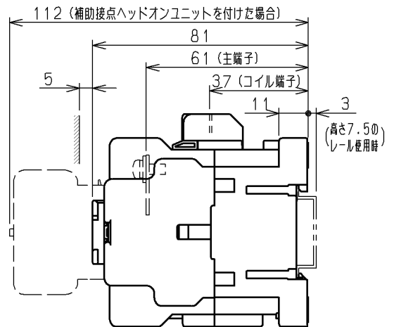
取付状態
