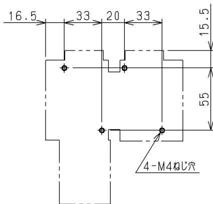
せん孔図
