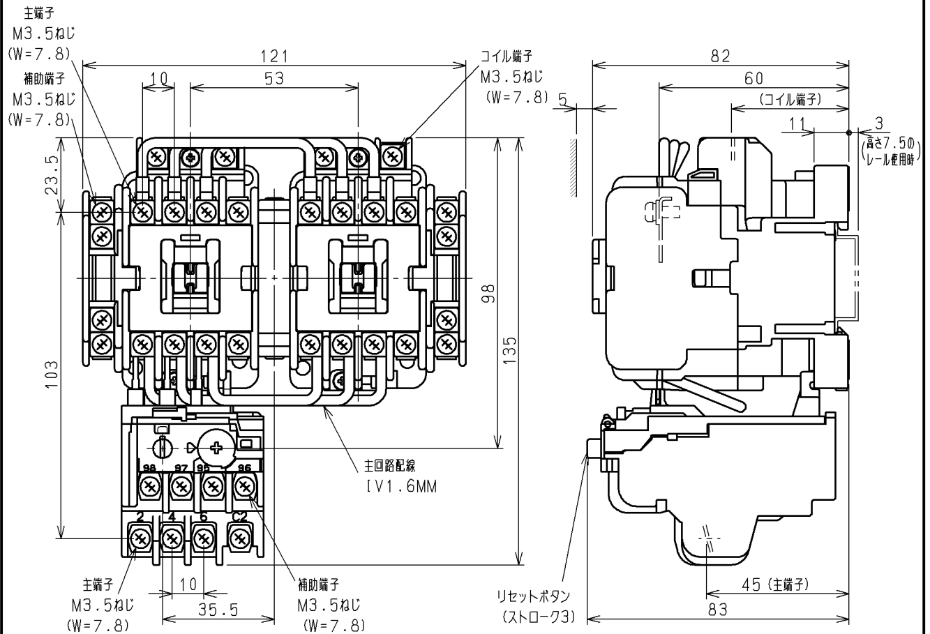
取付状態
