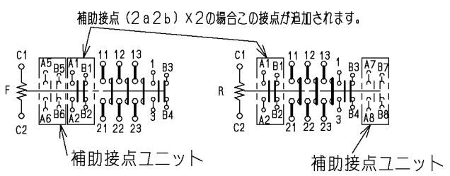
接点構成
