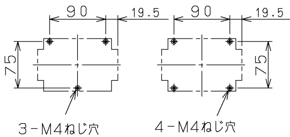
せん孔図
