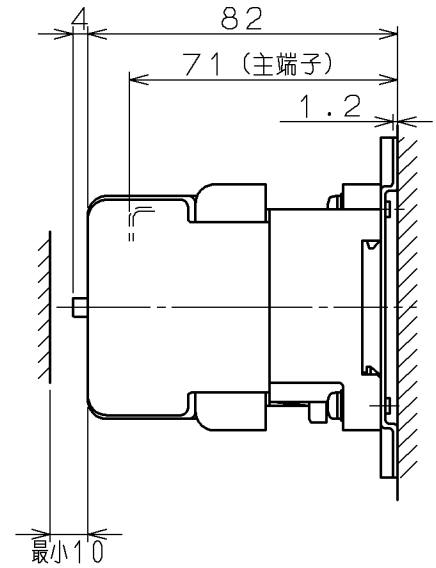
取付状態
