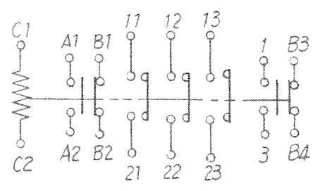
接点構成
