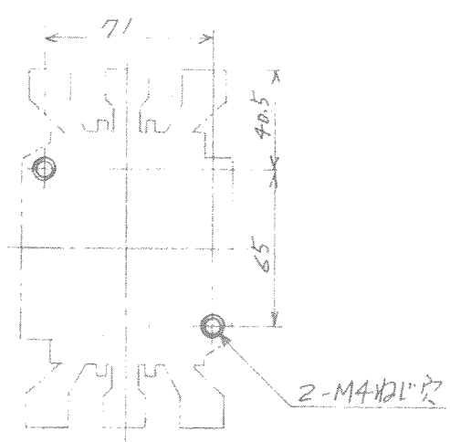
穴孔図
