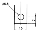
導帯加工図
