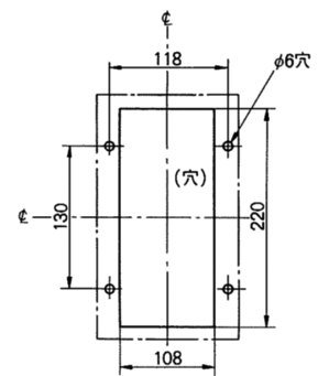
せん孔図
