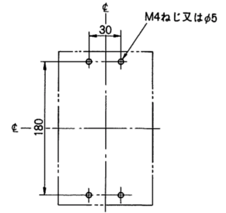
せん孔図
