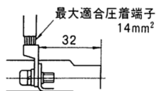
導帯, 圧着端子接続
