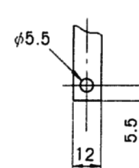
導帯加工図
