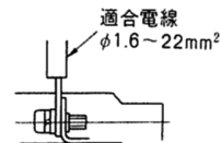
電線接続
