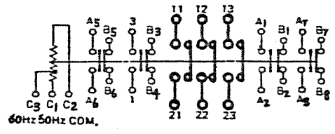
接点構成
