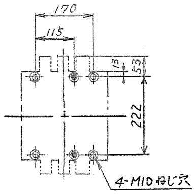
せん孔図
