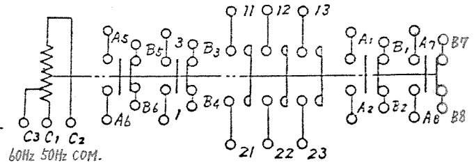
接点構成
