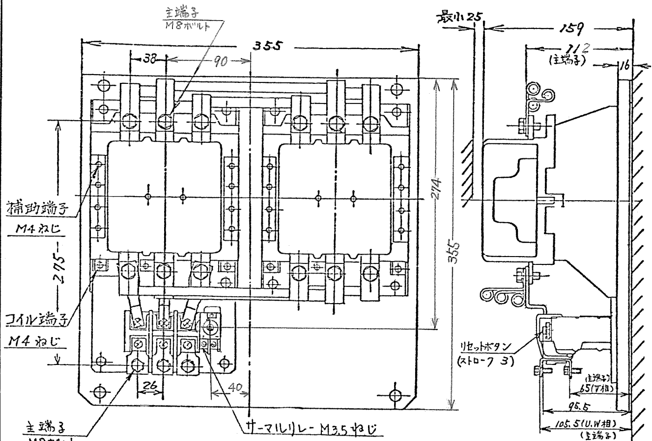
取付状態
