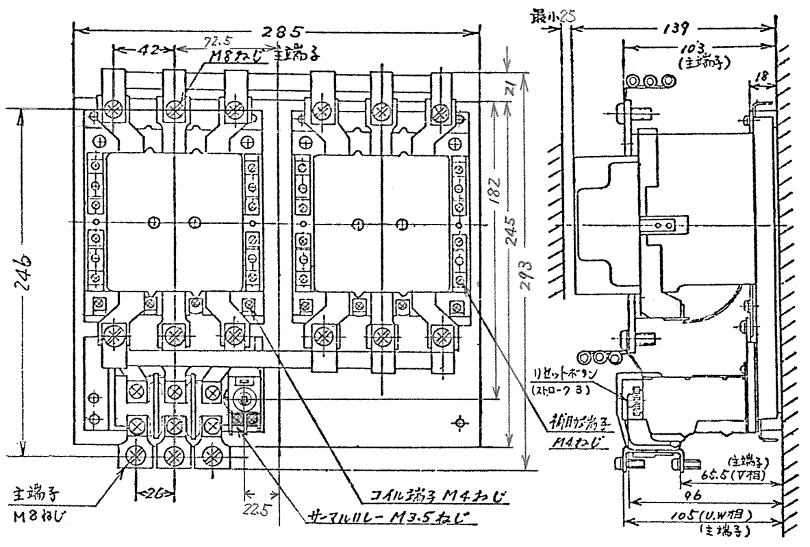
取付状態
