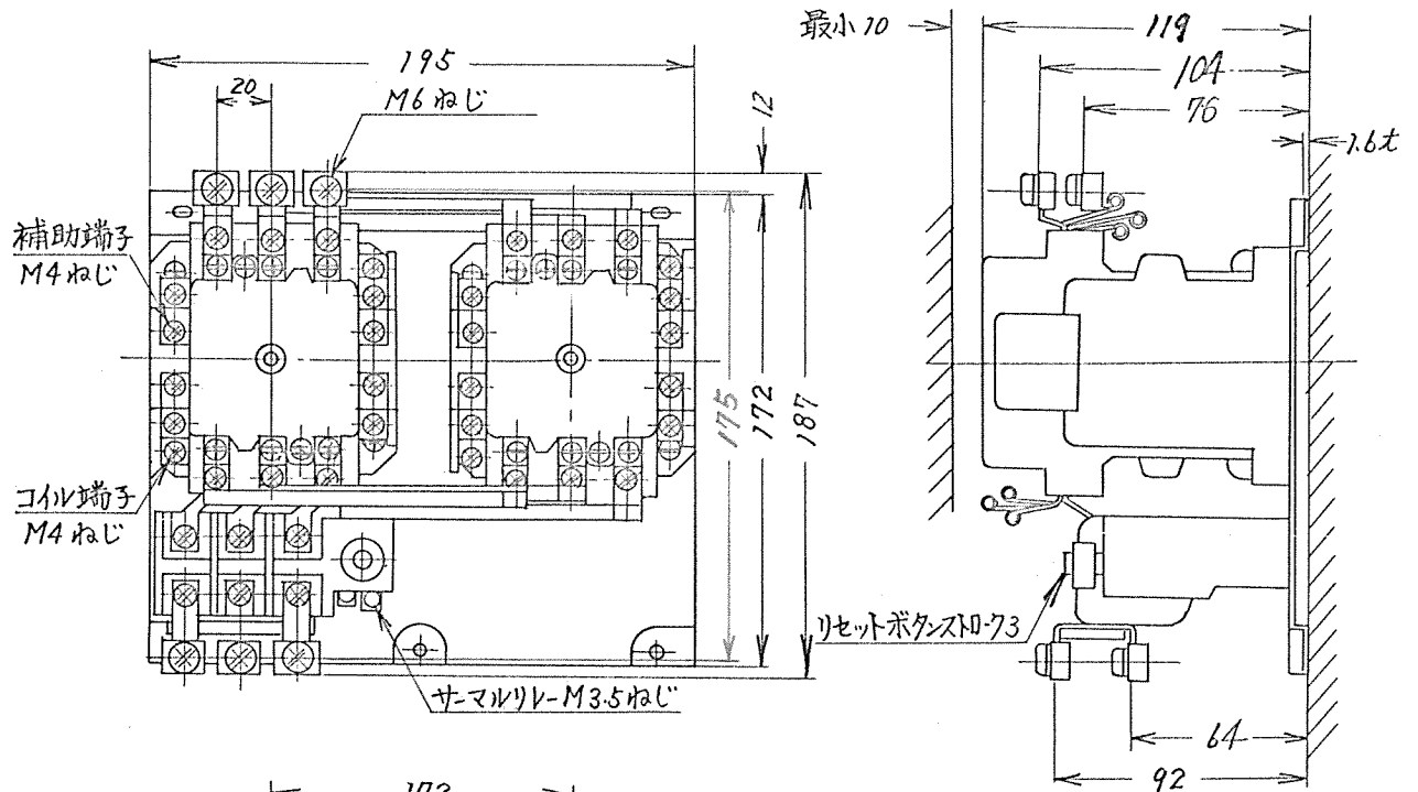
取付状態
