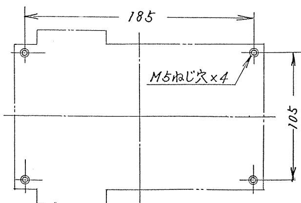
せん孔図
