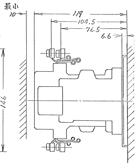
取付状態
