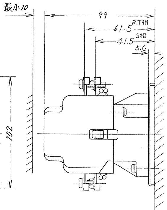
取付状態
