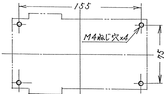
端子孔図
