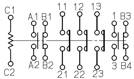
接点構成
