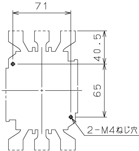
せん孔図
