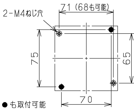
せん孔図
