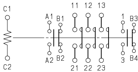
接点構成
