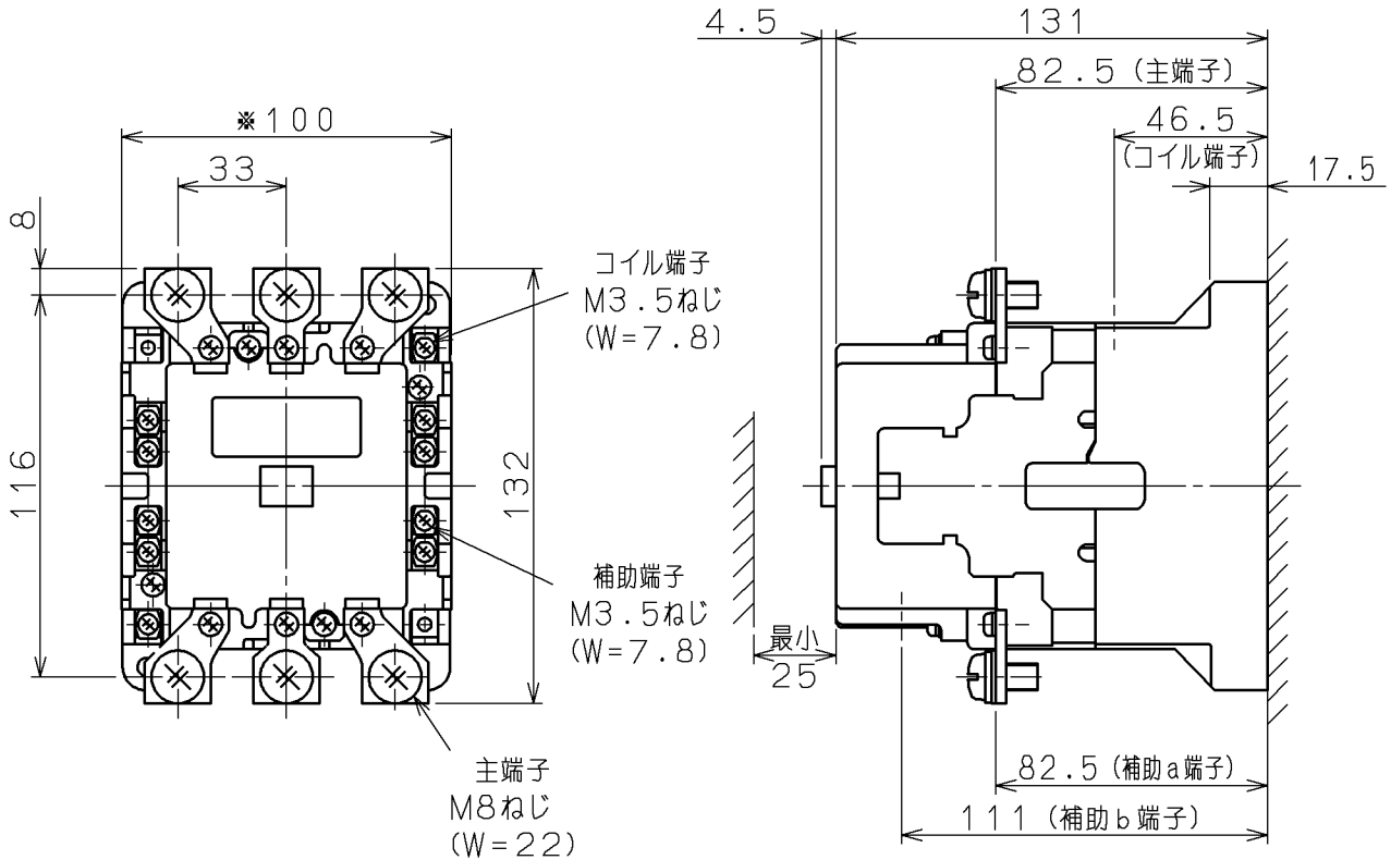
取付状態
