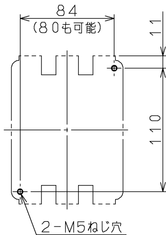
せん孔図
